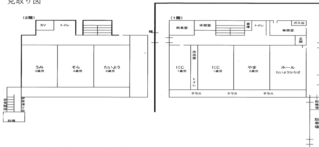
見取り図
