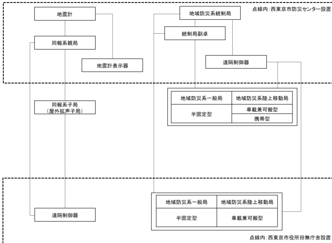
【市防災行政用無線局回線構成図】
