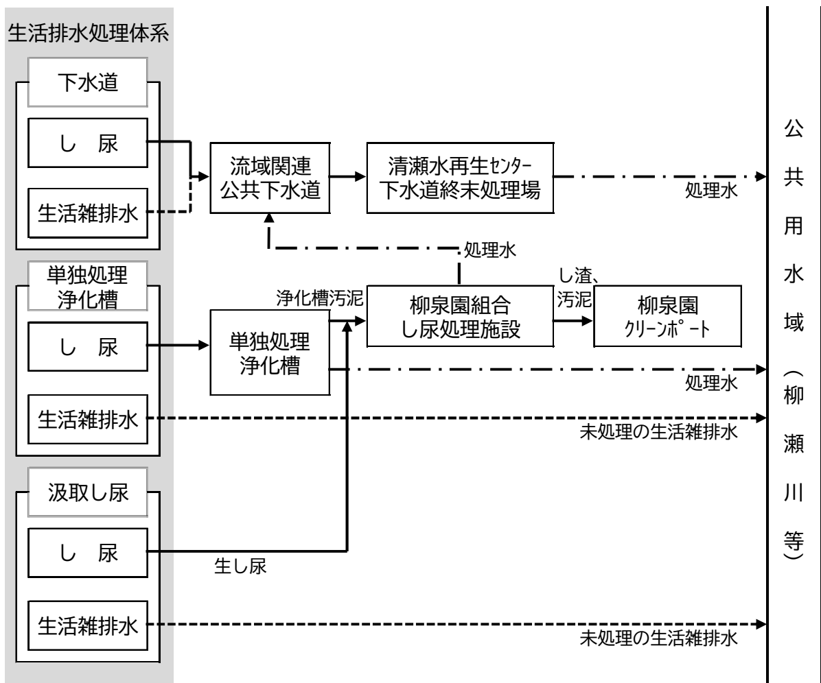
図 6-4 し尿処理施設の処理フロー
