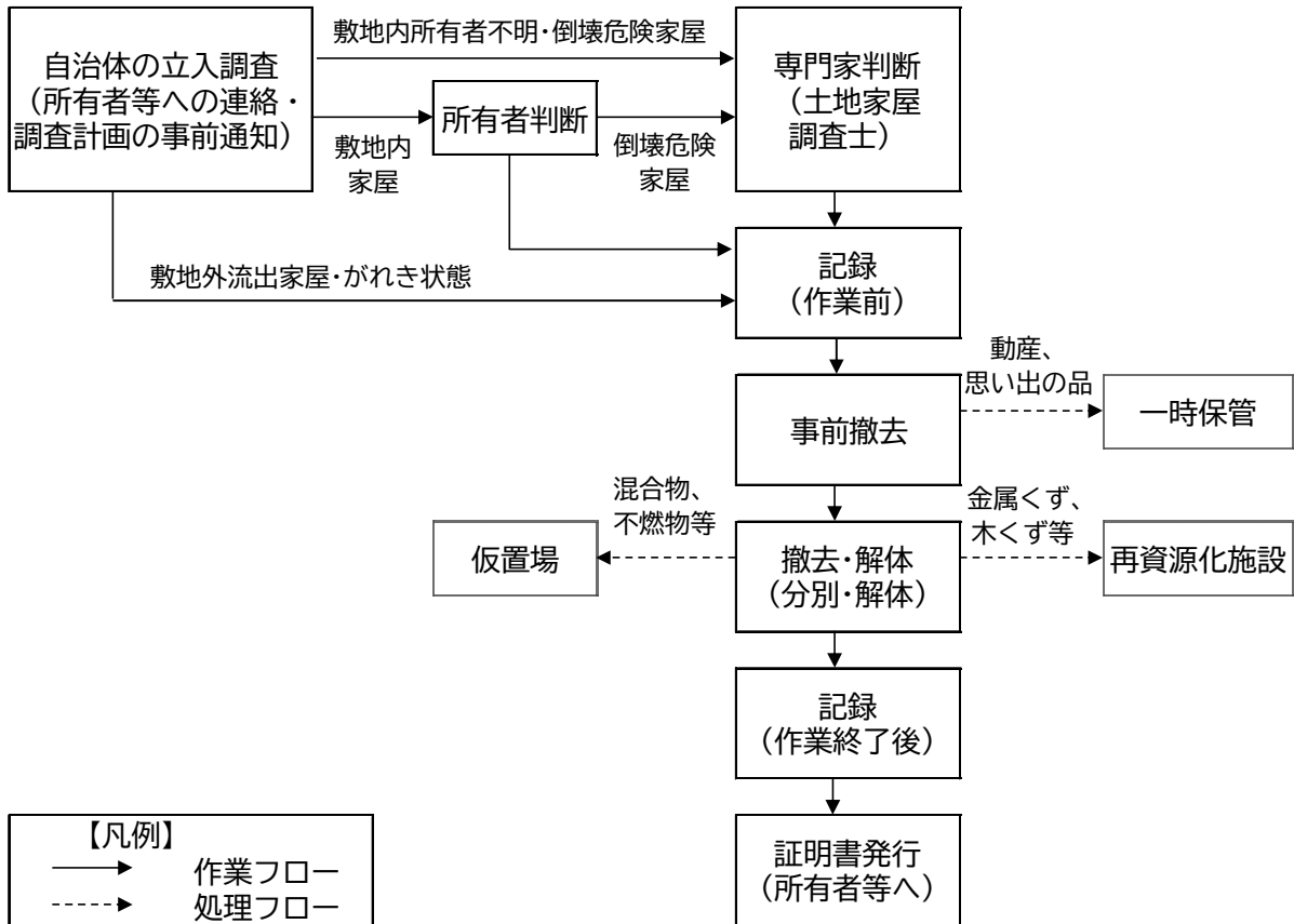
図 5-9 災害時の損壊家屋等の解体・撤去の手順
