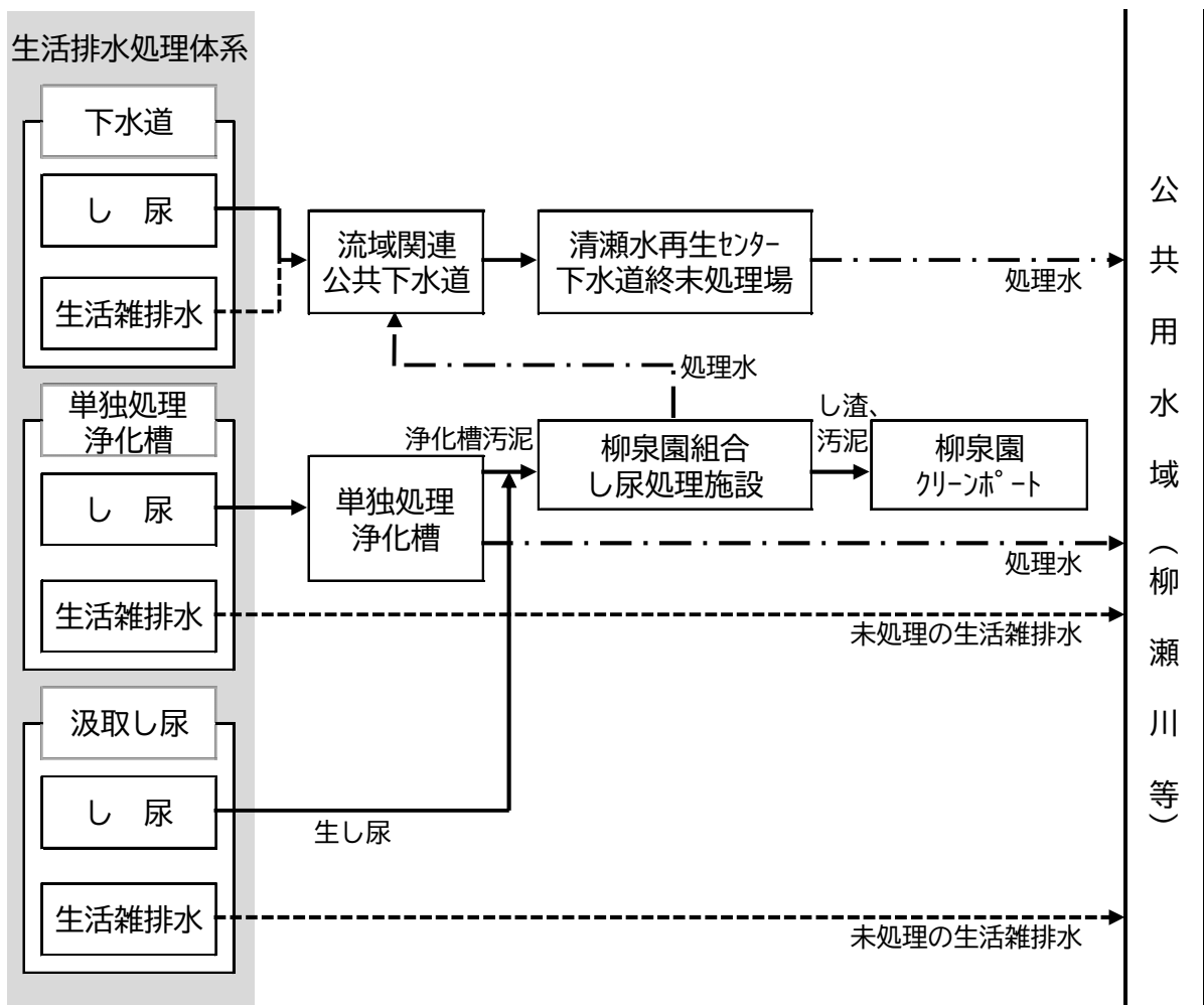
図 2-1 生活排水処理の体系
