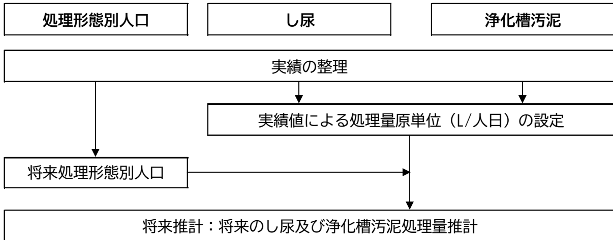
資料図 3 生活排水処理量推計フロー
