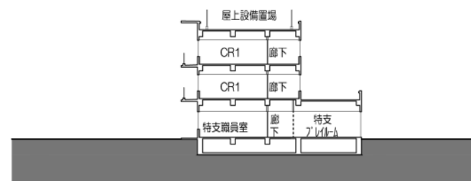
D-D'断面図
