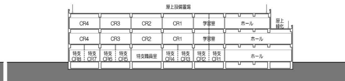
F-F'断面図
