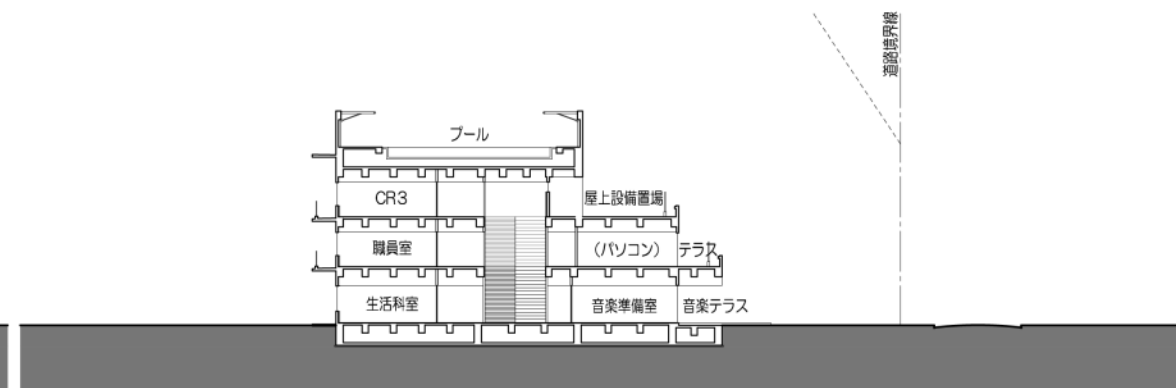
C-C'断面図
