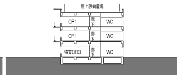
E-E'断面図
